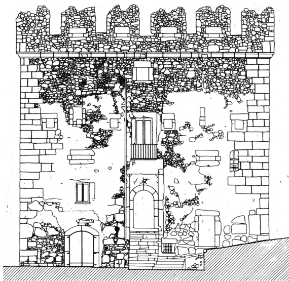
Fig. 10. Torre del mercato, prospetto del lato est (Valente 2000a, fig. a p. 37).
