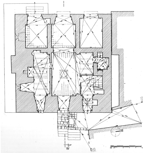
Fig. 15b. Torre del mercato: pianta del secondo livello (Valente 2000a, fig. a p. 35).
