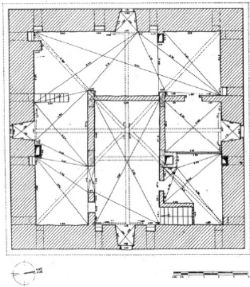
Fig. 15d. Torre del mercato: pianta del quarto livello (Valente 2000a, fig. a p. 36).
