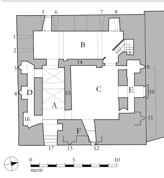
Fig. 15a. Torre del mercato: pianta del primo livello, 1-2, 5-8 feritoie orizzontali, 3-4, 9, 11-13, 16 bombardiere verticali, 10 porta tamponata, 14 parete est della galleria B, 15 muro di separazione fra gli ambienti A e C; 17 accesso attuale (disegno Rosario Claudio La Fata sulla base di Valente 2000a, fig. a p. 34);
