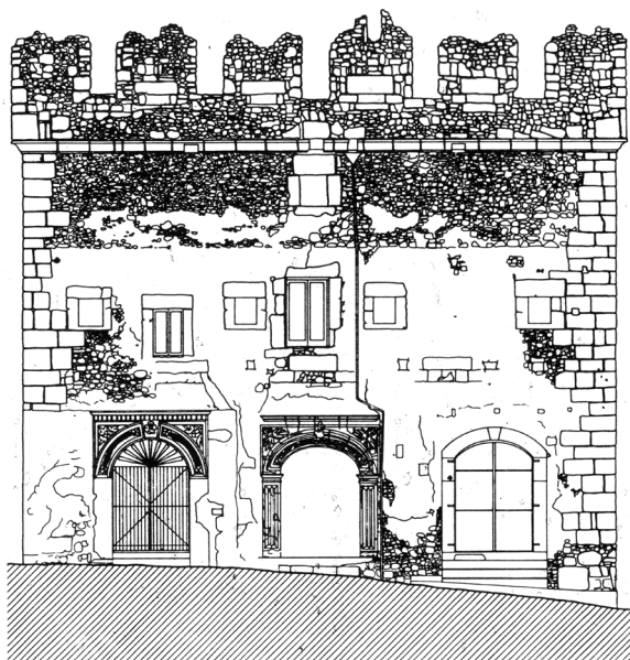
Fig. 8. Torre del mercato, prospetto del lato est (Valente 2000a, fig. a p. 39).
