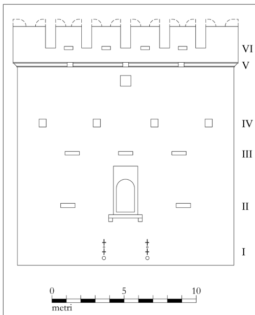
Fig. 11. Torre del mercato, prospetto del lato est con lo schema ricostruttivo del sistema difensivo (disegno R.C. La Fata sulla base di Valente 2000a, fig. a p. 37).
